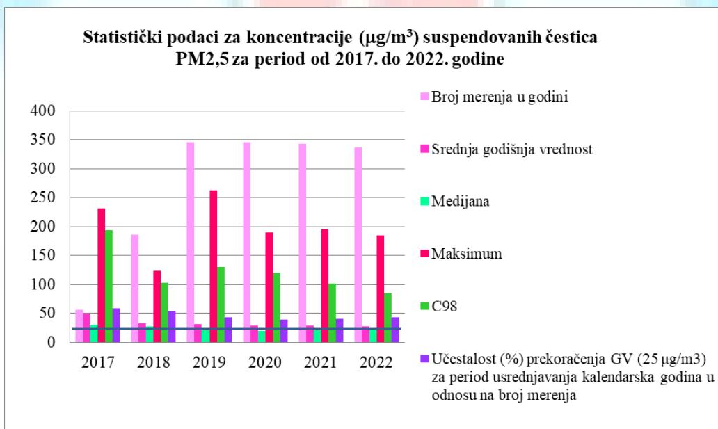
Grafikon 10. Prikaz broja merenja i srednjih godišnjih vrednosti izmerenih koncentracija [ \mu\text{g}/\text{m}^3 ] i ostalih statističkih podataka za suspendovane čestice PM 2,5 u vazduhu za 2022. godinu u poređenju sa 2017., 2018., 2019., 2020. i 2021. godinom na mernim mestima: Gradska Bolnica Subotica (period od 2017. do juna 2018. godine) i osnovna škola “Sonja Marinković” Mala škola u Subotici (period od jula 2018. do kraja 2022. godine), ( GV je 25 \mu\text{g}/\text{m}^3 za period usrednjavanja kalendarska godina)
