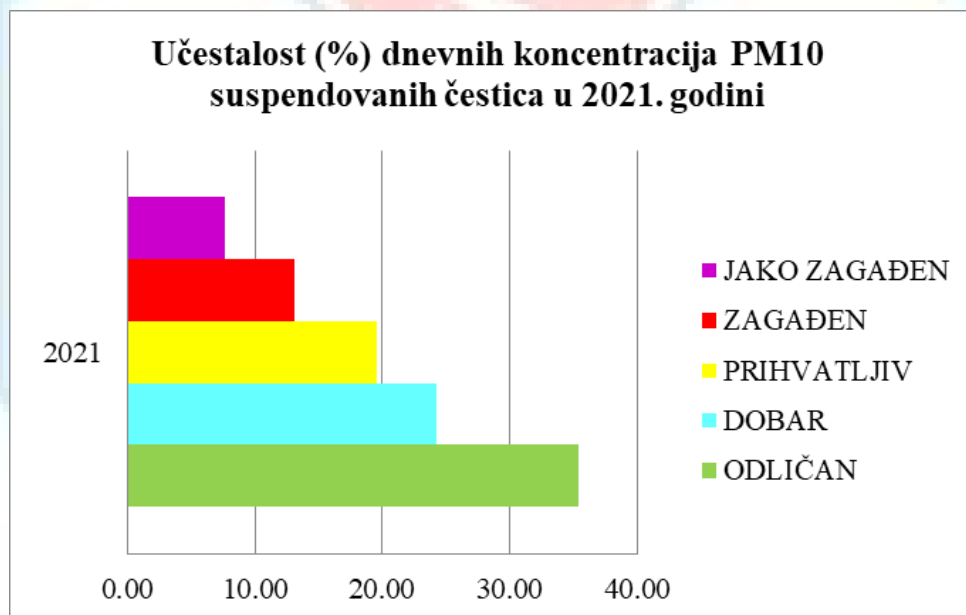
Grafikon 7. Kvalitet vazduha - učestalost (%) klasa kvaliteta vazduha po Indeksu kvaliteta vazduha SAQI_11 određenih na osnovu dnevnih vrednosti kocentracija suspendovanih čestica PM10 u vazduhu u 2021. godini na mernom mestu osnovna škola “Sonja Marinković” Mala škola u Subotici
