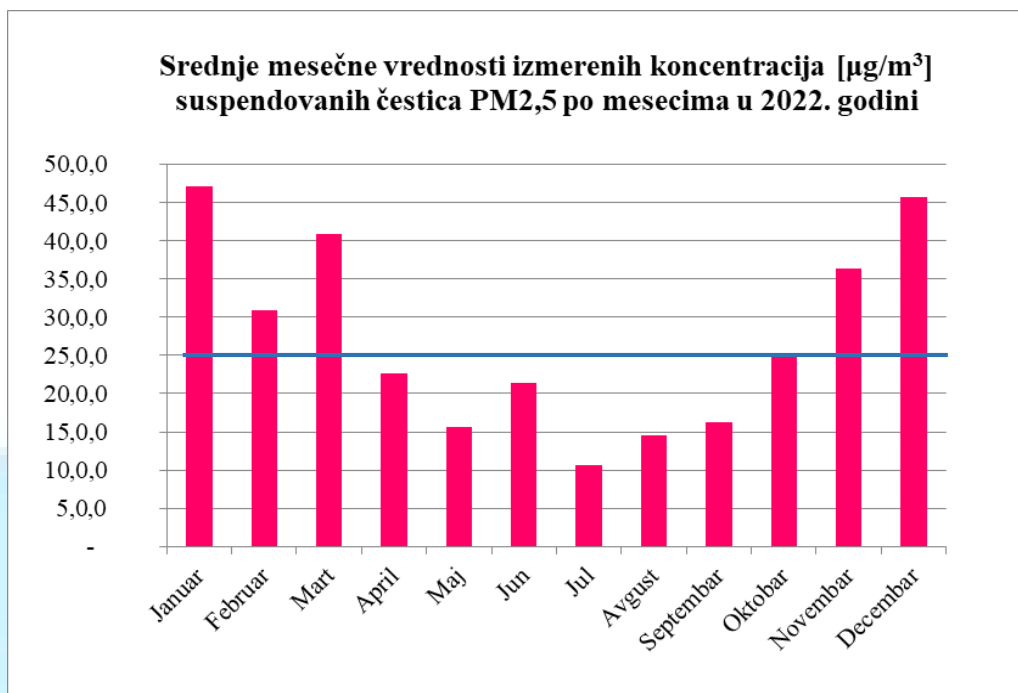
Grafikon 9. Srednje mesečne koncentracije suspendovanih čestica PM 2,5 u vazduhu na mernom mestu osnovna škola “Sonja Marinković” Mala škola u Subotici po mesecima u 2022. godini ( GV je 25 \mu\text{g}/\text{m}^3 za period usrednjavanja kalendarska godina)
