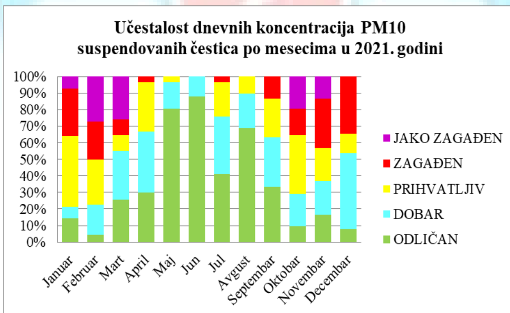
Grafikon 5. Kvalitet vazduha - učestalost (%) klasa kvaliteta vazduha po Indeksu kvaliteta vazduha SAQI_11 određenih na osnovu dnevnih vrednosti koncentracija suspendovanih čestica PM10 u vazduhu po mesecima u 2021. godini na mernom mestu osnovna škola “Sonja Marinković” Mala škola u Subotici
