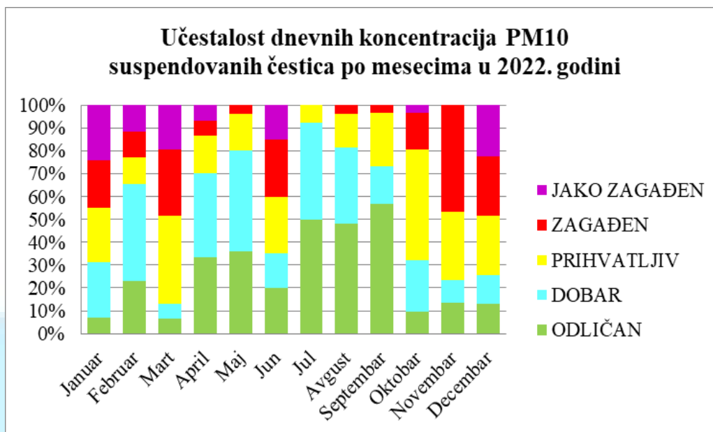
Grafikon 4. Kvalitet vazduha - učestalost (%) klasa kvaliteta vazduha po Indeksu kvaliteta vazduha SAQI_11 određenih na osnovu dnevnih vrednosti koncentracija suspendovanih čestica PM10 u vazduhu po mesecima u 2022. godini na mernom mestu osnovna škola “Sonja Marinković” Mala škola u Subotici
